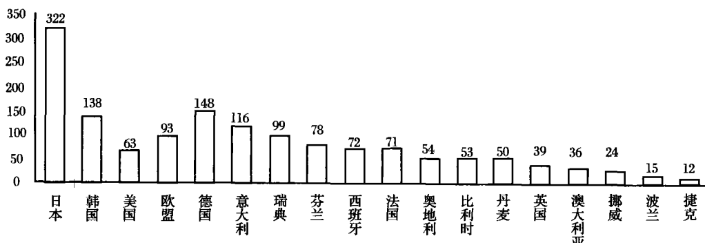
图 1 2003年制造业中每 1万名雇员拥有工业机器人的数量
