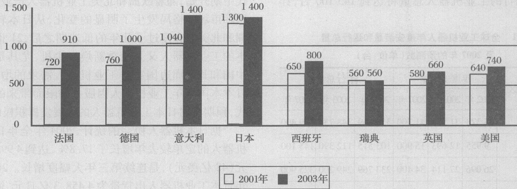
图 2 2001和 2003年,汽车制造业中每 1万名产业工人拥有的工业机器人数量(单位:台)
